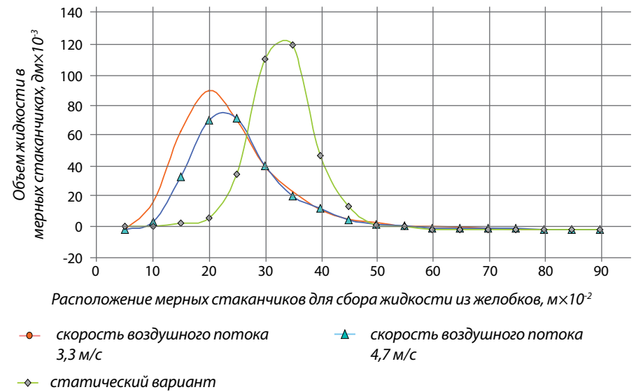
Рис. 4. Распределение жидкости в продольном направлении в статическом варианте и при разных скоростях воздушного потока
