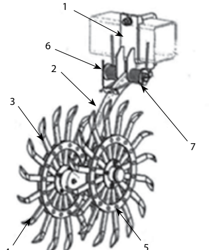
Рис. 2. Секция рабочих органов бороны БРН-5,8: 1 — кронштейн; 2 — стойка; 3 — кулиса; 4, 5 — диск ротационный игольчатый; 6, 7 — пружина стабилизирующая
