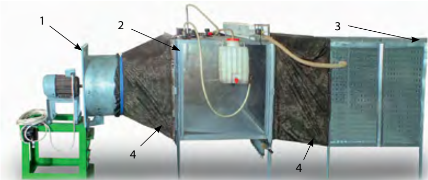
Рис. 2. Общий вид стендового оборудования для моделирования технологий распылителей штанговых опрыскивателей: 1 — модуль для создания воздушного потока с требуемыми характеристиками; 2 — узел для распыления жидкости и улавливания оседающих капель в поперечном и продольном направлении; 3 — модуль с отверстиями для снижения скорости воздушного потока и распределения мелкодисперсного аэрозоля; 4 — кожух соединительный
